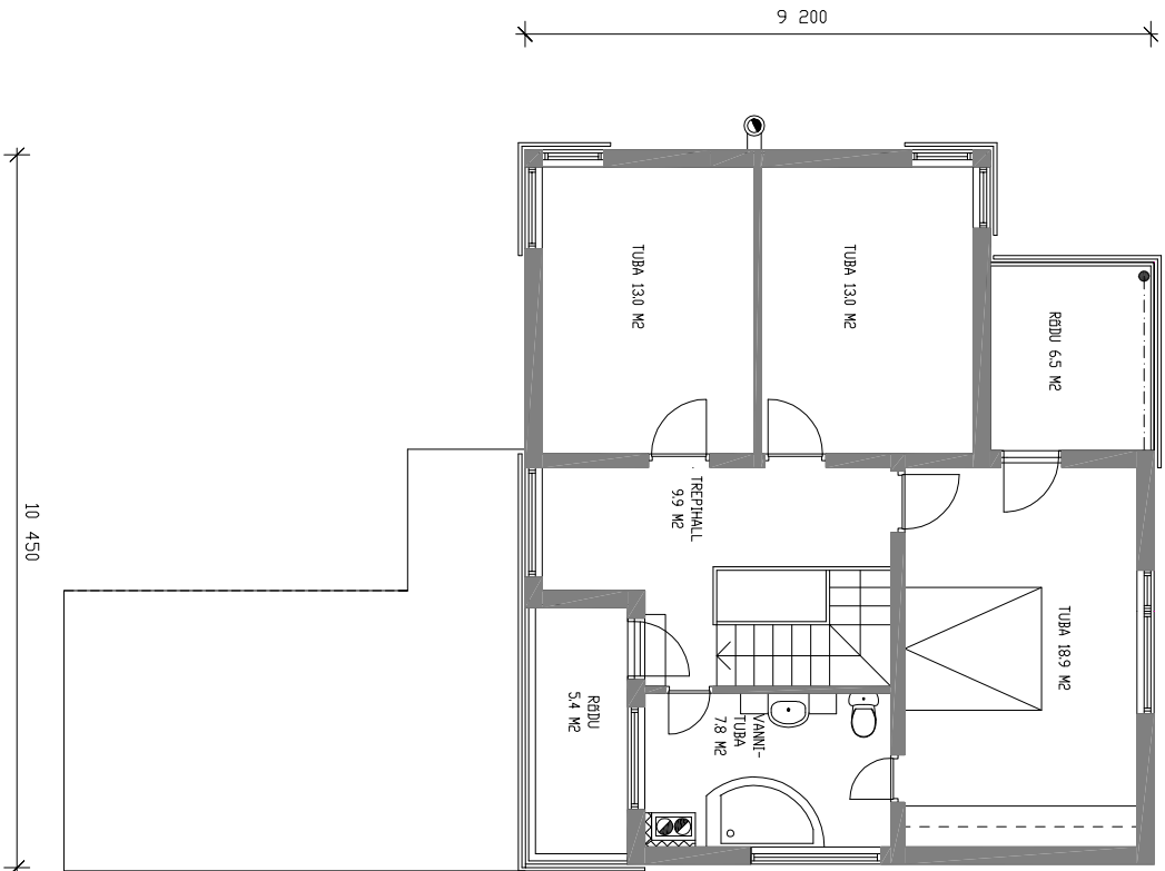
2-KORRUSE PLAAN
